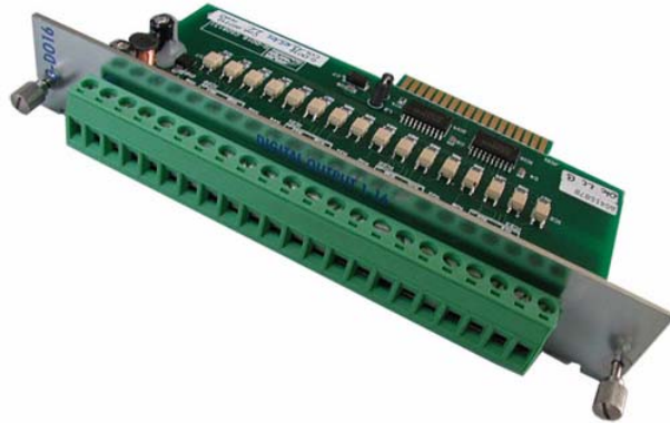
Figura 1 : Scheda G-DO16 - 16 uscite digitali
